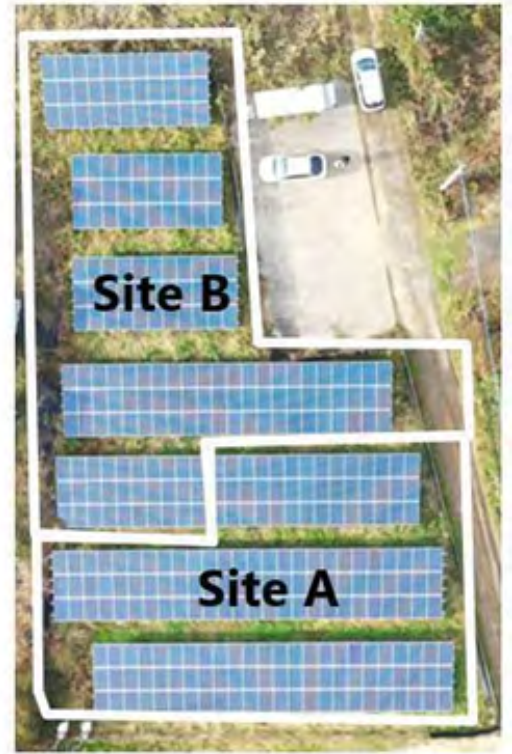
サイトAおよびサイトBはお互いに隣接した低圧サイトです。Mr.DreamはまずサイトAをソーラーエッジでりパワリングすることとしました。下図は、サイトAとサイトBの4年間の発電(10月から12月のみ)を比較したものです。
